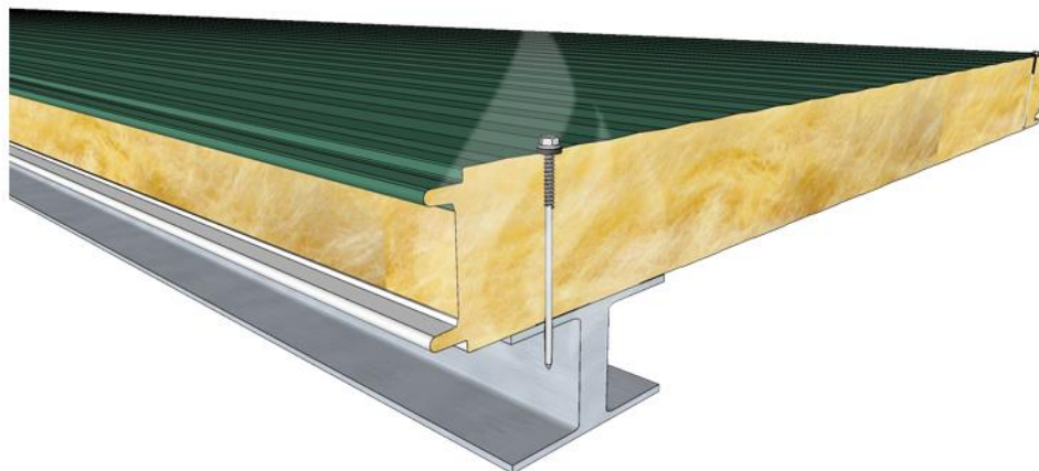
Sendvičový panel z minerálnej vlny, tex samorezná skrutka a ocelový nosník ( I profil)
